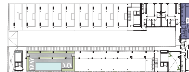
PLANTA TERCERA
